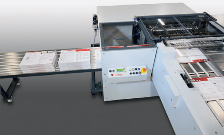
Kontinuierliche Stapelauslage von Sätzen auf Band (mit Überlaufschutz).
